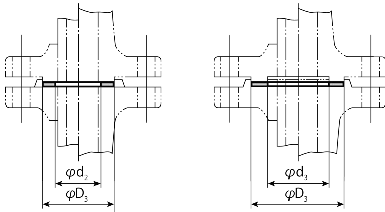
MF(非金属平形)ガスケット / TG(非金属平形)ガスケットの形状・寸法
